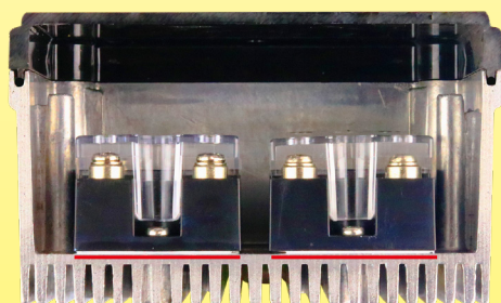
Ejemplo de instalación de relés de estado sólido en una carcasa de aluminio de Ultimheat (compueste térmico en rojo).
